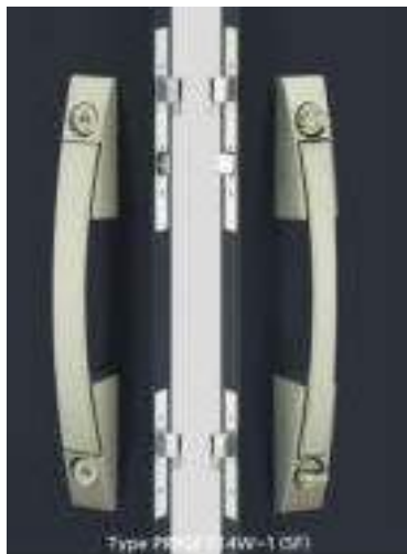
Model/ Mã số PGF714W(SF) Material Die-cast aluminum Chất liệu Nhôm đúc Finishes Stainless color painted Hoàn thiện Sơn chống gỉ Size (mm) 51x438 mm(RxD) Application 36-45mm door thickness range Ứng dụng Độ dày cửa 36-45mm
