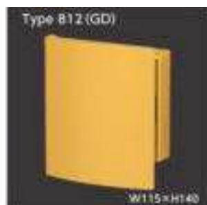
Model/ Mã số Type 812(GD) Material Aluminum Finishes Semi-gloss satin gold color anodized aluminum Size (mm) 140x115 mm(RxD) Application 33-66 mm door thickness Ứng dụng Độ dày cửa 33-66mm
